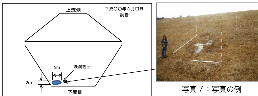
図4：変状箇所のスケッチ
