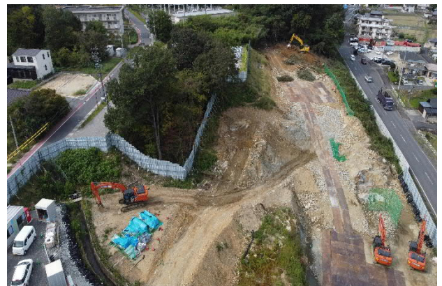
大井非常口ヤード全景
