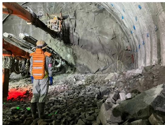
トンネル掘削作業状況 （発破装薬状況）
