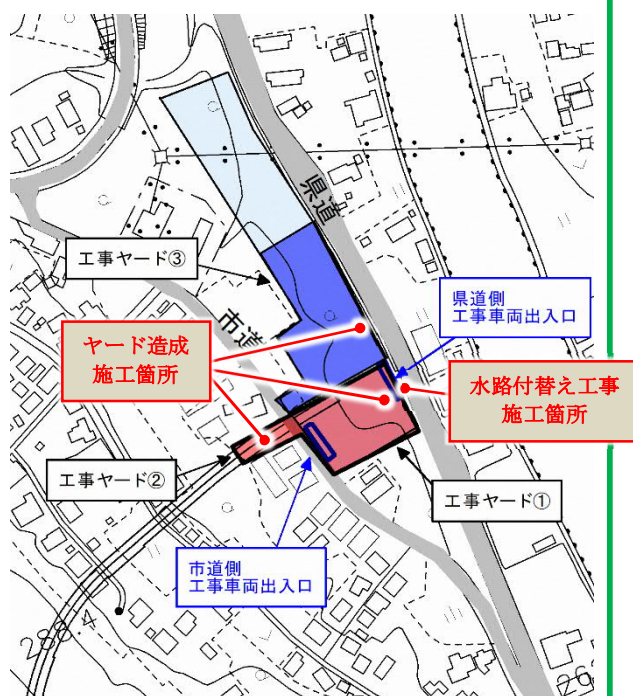
大井非常口ヤード全景（模式図）
