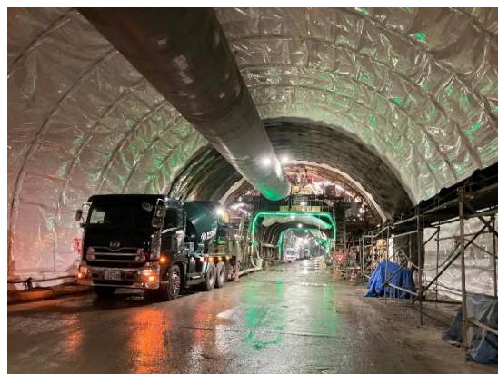
覆工コンクリート工作業状況 （打設状況）
