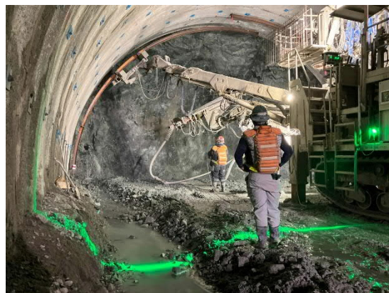
トンネル掘削作業状況 （吹付コンクリート状況）
