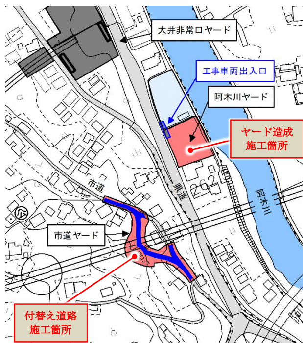
付替え道路施工ヤード全景（模式図）
