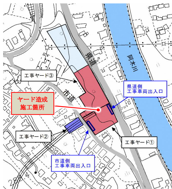
大井非常口ヤード全景（模式図）
