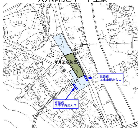
大井非常口ヤード全景
