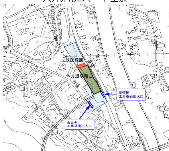
大井非常口ヤード全景
