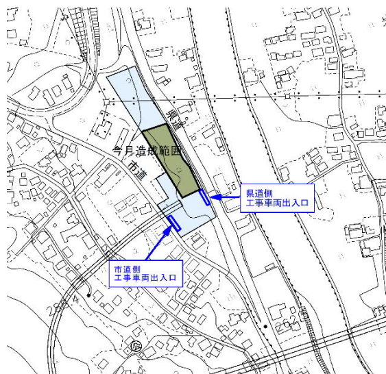
大井非常口ヤード全景
