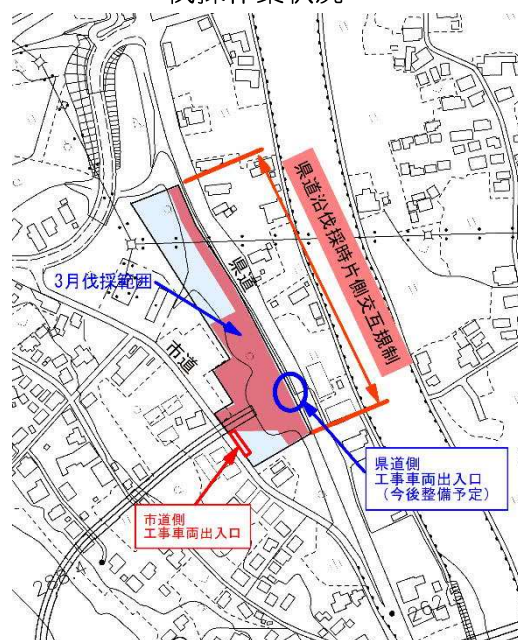
平面図
