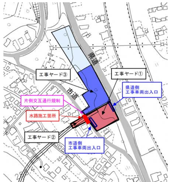
大井非常口ヤード全景
