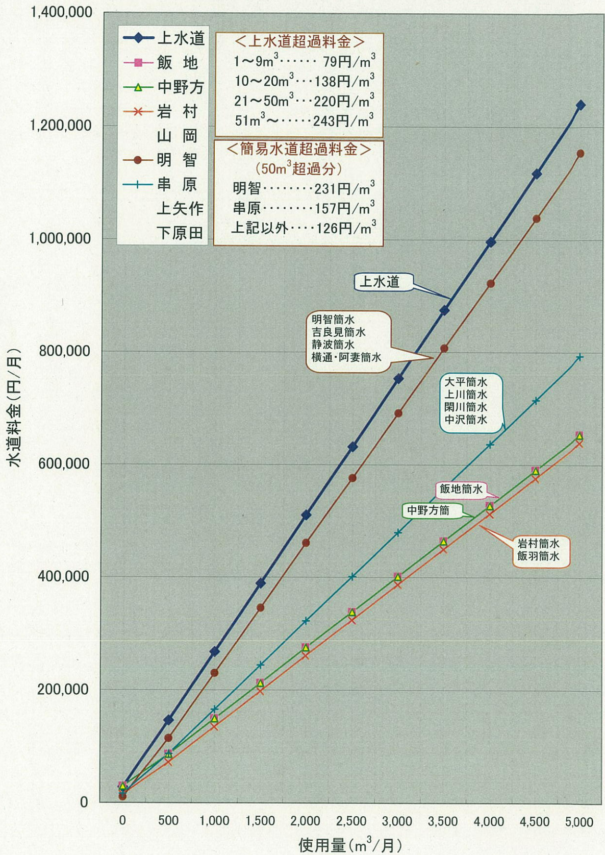
水道料金比較表(口径75mm)
