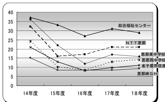
【二酸化硫黄】
