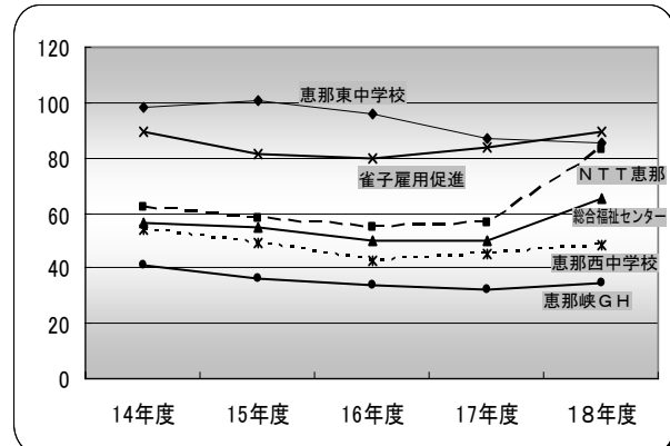
【二酸化窒素】
