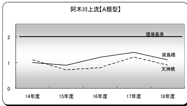
[図 3-2-1] BOD75%値の経年変化
