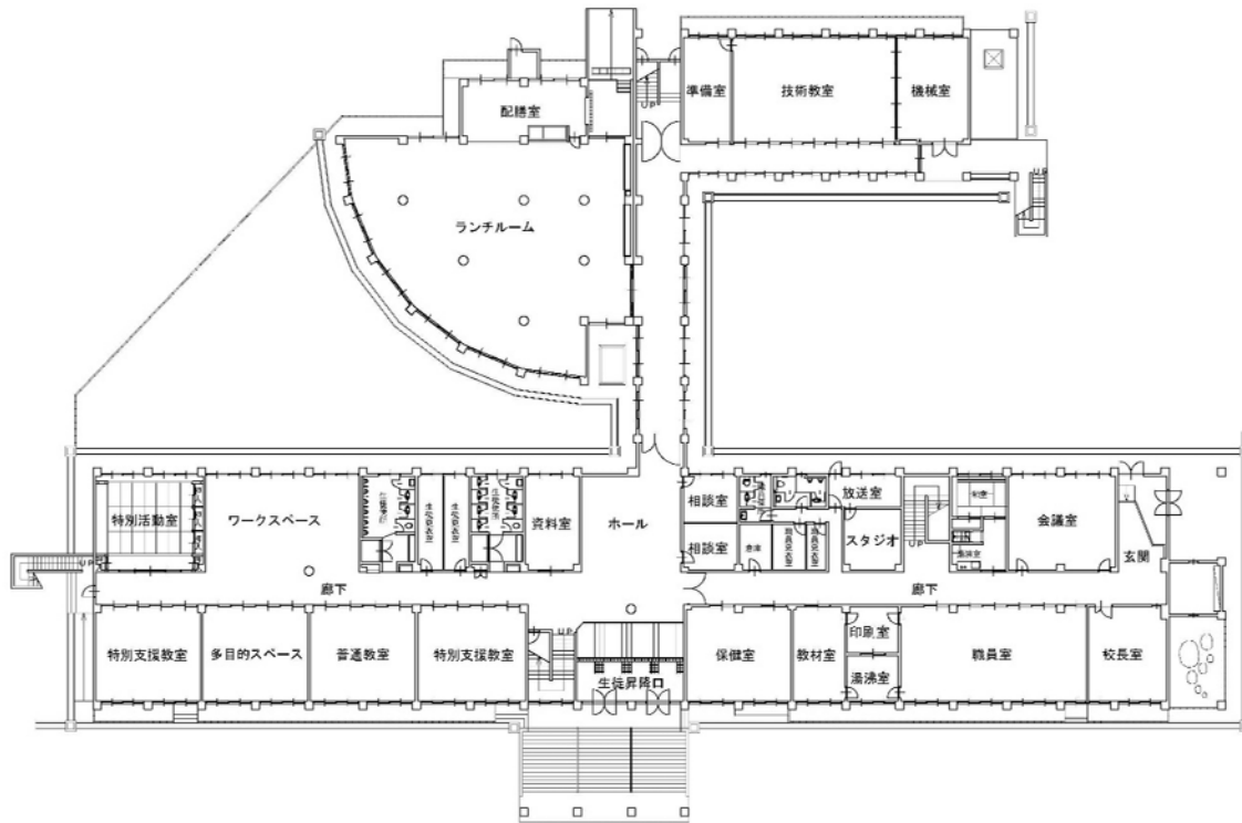
山岡中学校 1階平面図
